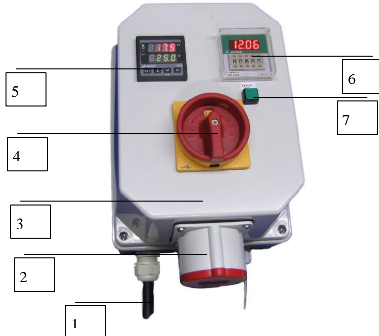
Gesamtansicht Regler RT2-51/511 – (Beispielhafte Abb)
