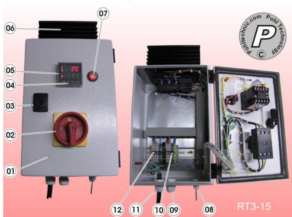
Gesamtansicht Regler RT3-15-SSR (Abb ähnl.)
