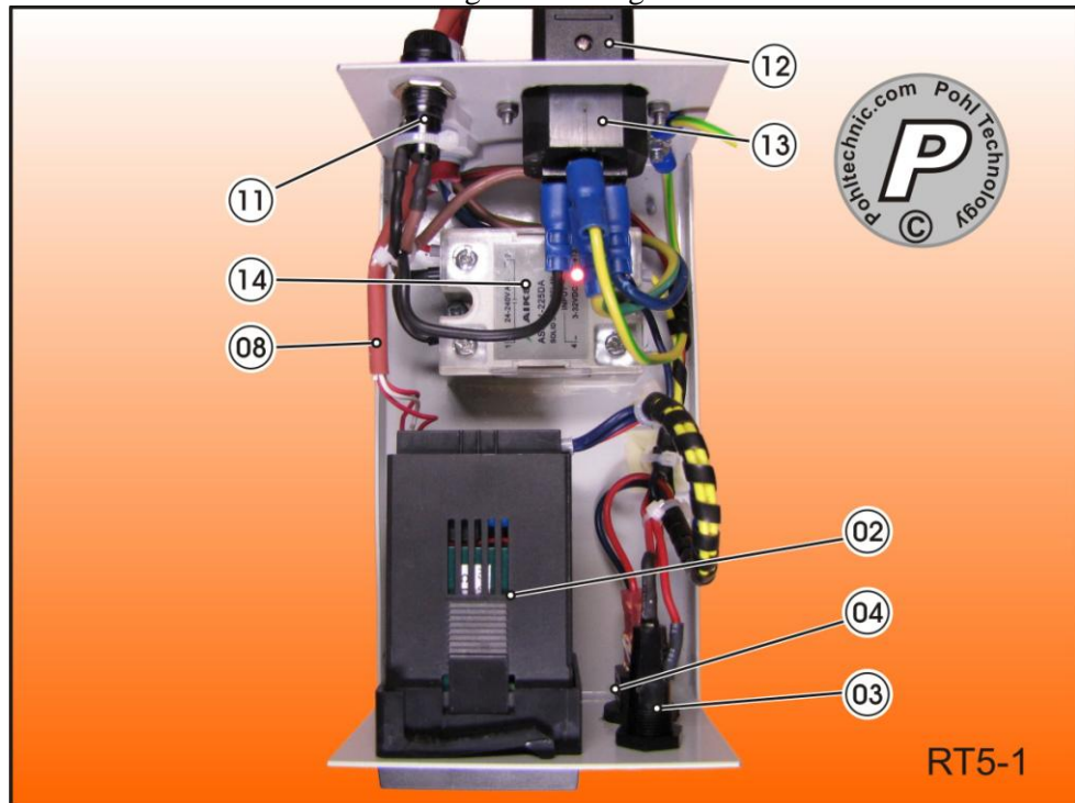
Verdrahtungsansicht Regler RT5-1
