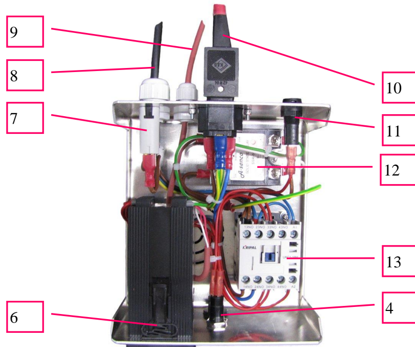
Gesamtansicht Regler RT5-24 Abb. ähnl.)
